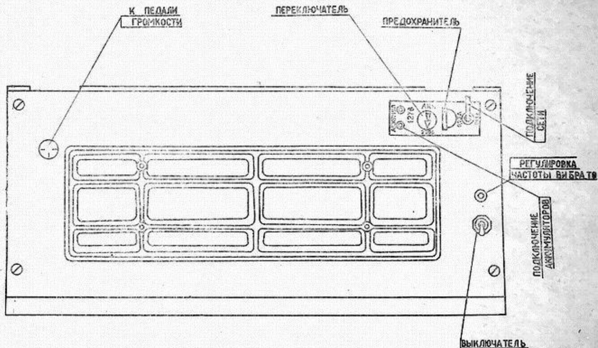
Рис 4 Вид снизу
